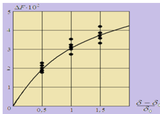
Рис. 1. Увеличение коэффициента замещения отопительной нагрузки с изменением толщины теплоаккумулирующей стенки.
