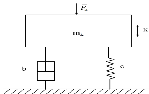
Рис.1. Расчетная схема колебаний колосника на резиновых опорах
