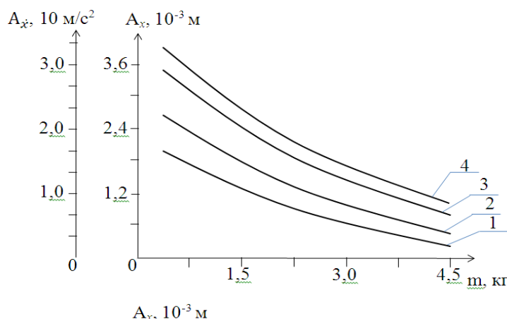
Рис.3 Графические зависимости изменения амплитуды перемещения и скорости колебаний колосника от вариации коэффициента жесткости упругой резиновой втулки колосника
