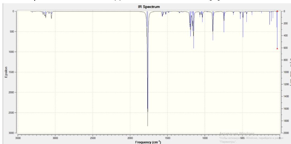
Рисунок 2. ИК-спектроскопия молекулы бисаланината железа
