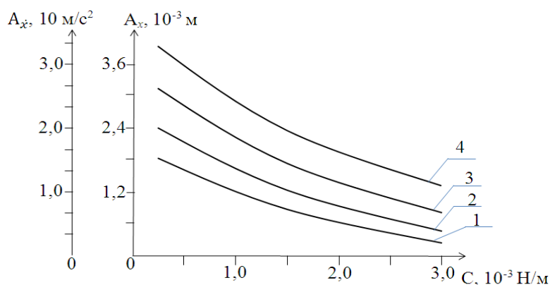
Рис. 2. Графические зависимости изменения амплитуды колебаний перемещений и скоростей колосника на резиновых подушках от технологической нагрузки хлопка-сырца
