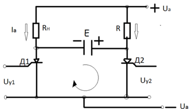
Рис. 2. Схема тиристорного реле.
