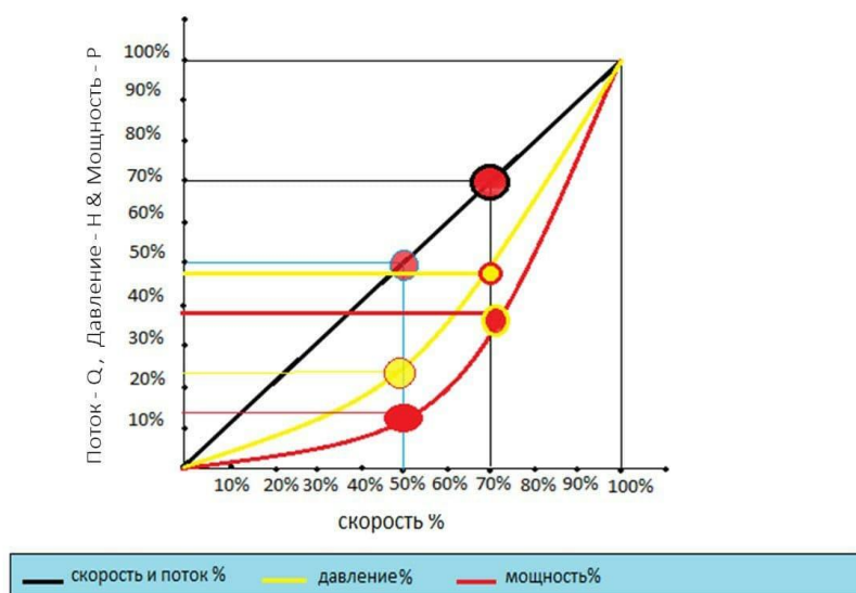
Рис.4.График изменения основных параметров центробежного насоса при уменьшении скорости на 30% и на 50%.
