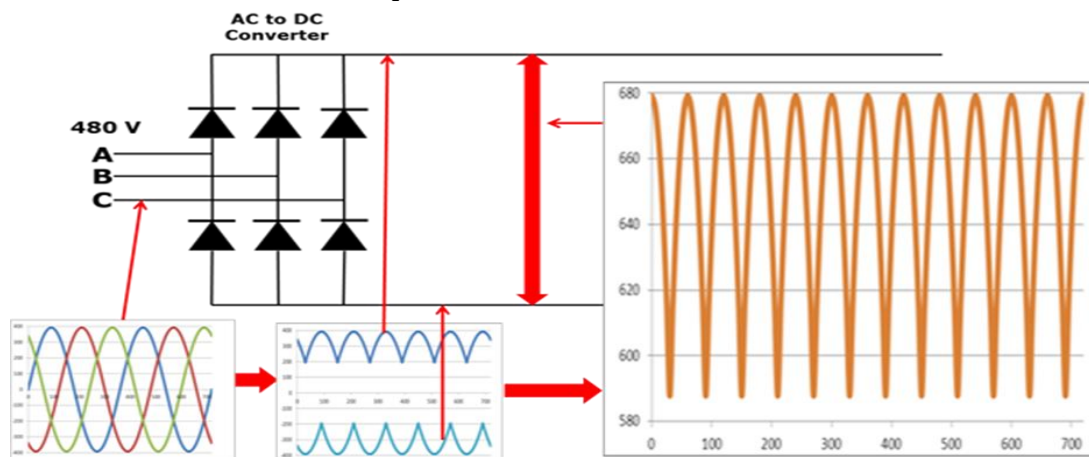
Рис 6 Схема AC\DC преобразователя в системе VFD
