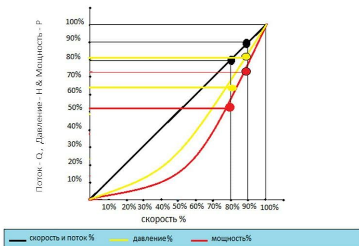
Рис.5. График изменения основных параметров центробежного насоса при уменьшении скорости на 10%( f=45Гц ) и на 20%( f=40Гц ).
